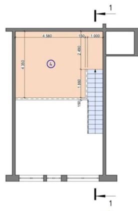
Монтажный план антресоли нежилого помещения на отм. +2.280, М 1:100
