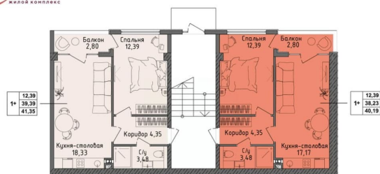
Секция 8 Этаж 1
