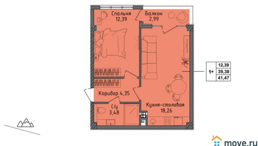
Секция 10 Этаж 2
