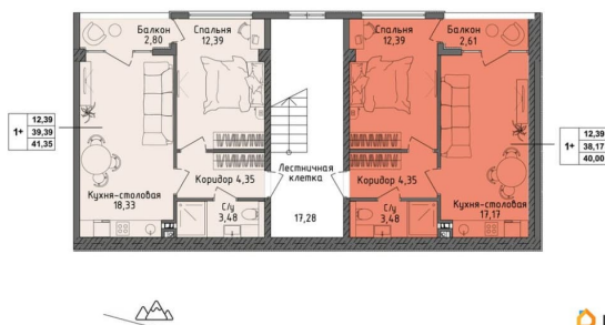
Секция 5 Этаж 1
