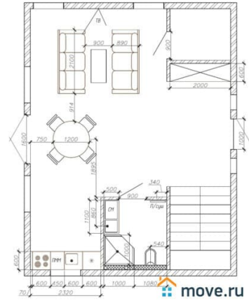
Дом №3, 1 этаж План с расстановкой мебели
