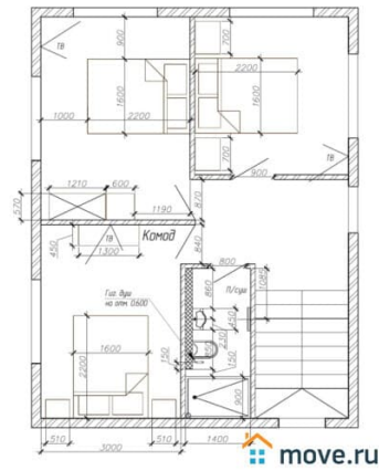
Дом №2, 2 этаж План с расстановкой мебели
